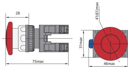
Кнопка «грибок» Ø 40 мм с пружинным возвратом
