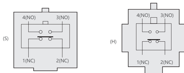
Рис. 1. Расположение контактов
